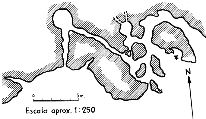
Croquis en planta de la cueva de Marizulo en Urnieta
