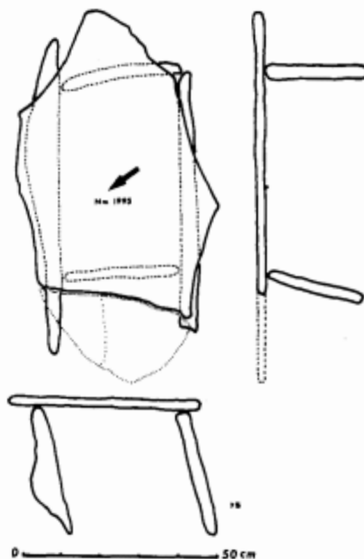
Figure 2.- Vue en plan, face, et profil du caisson central. En pointillé fin. l'extrémité NO. du couvercle brise en deux fragments.
