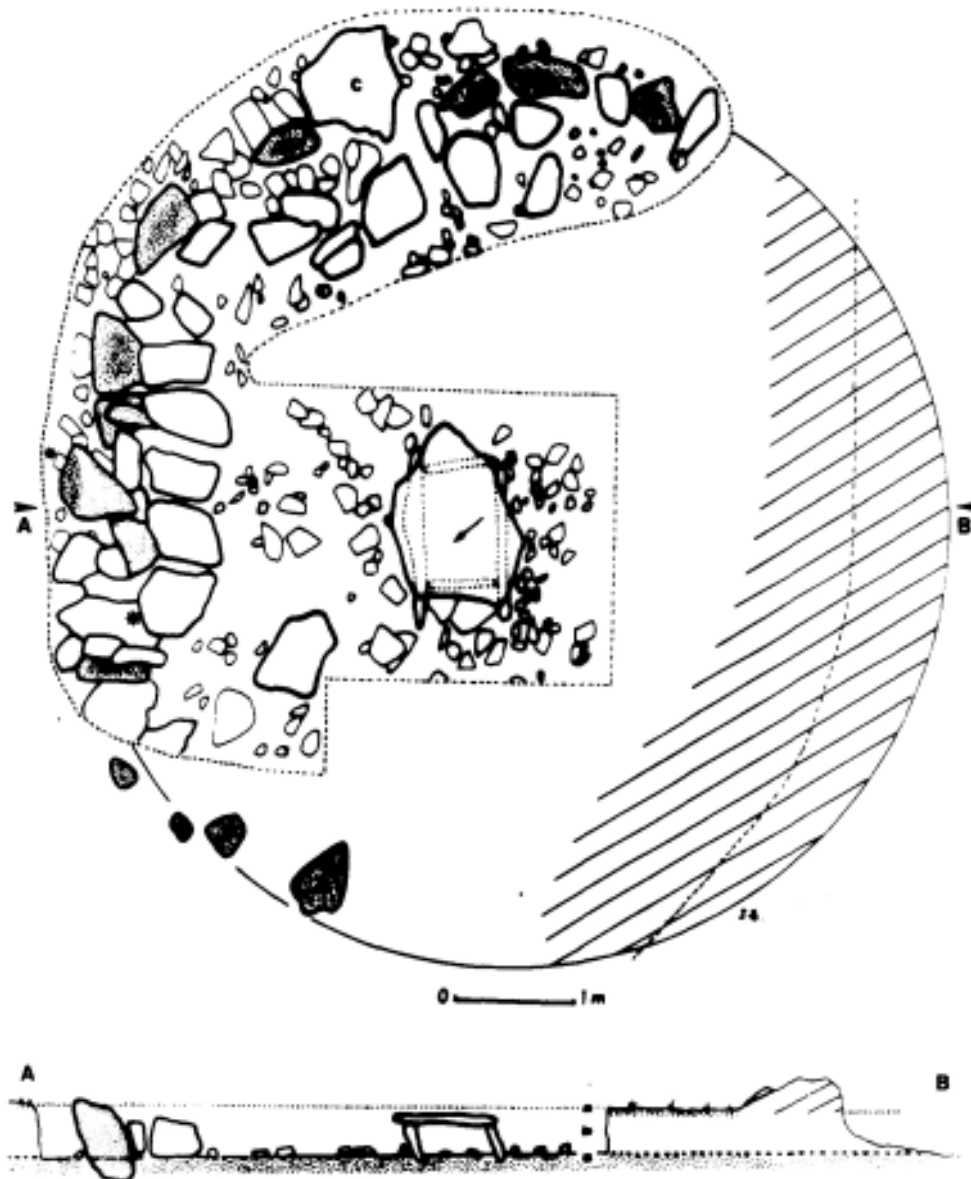
Figure 1.- Plan et coupe de Mendizabale 7
