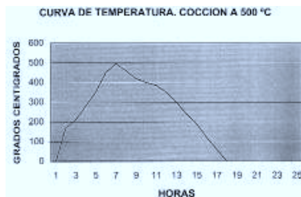
Figura 13.1. Curva de temperatura de cocción de las muestras experimentales.
