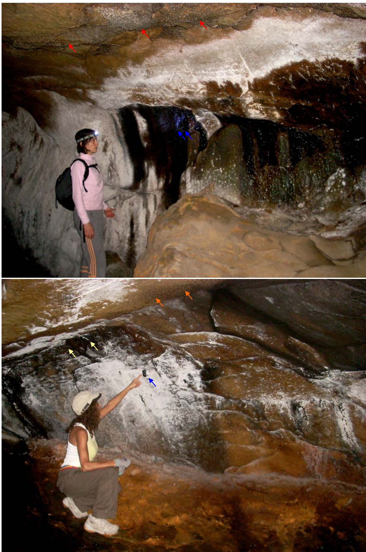
Figura 1. La cueva Jaizkibel 07 (JK-07 Green Cave) posee una notable diversidad de espeleotemas. En la imagen superior pueden apreciarse recubrimientos blancos de silicatos de aluminio amorfos, recubrimientos negros de hematita y magnetita con tonos metálicos (flechas azules) y pequeñas espeleotemas de yeso (flechas rojas). En la imagen inferior se aprecian ejemplos de vermiculaciones arcillosas (flechas naranja), espeleotemas negras de hematita y magnetita (flechas blancas), algunas de ellas formando estalactitas de hasta 4 cm (flecha azul). Los colores negros más intensos sugieren la presencia de óxidos-hidróxidos de manganeso, en pequeñas cantidades.
