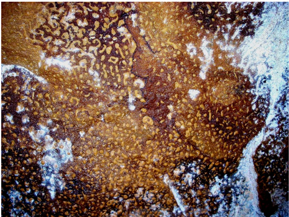
Figura 2. Ejemplos de vermiculaciones arcillosas, de tipos jeroglífico y motas de leopardo, en Green Cave JK-07. El material de las vermiculaciones, en relieve positivo, está compuesto de mica-illita, con trazas de hematita.
