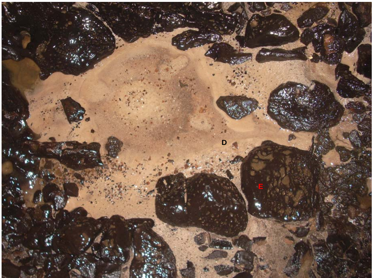
Figura 6. Otros ejemplos en la cueva Jaizkibel 07. En la imagen superior, espeleotemas de hematita y magnetita formando pequeñas estalagmitas parietales de colores ocre-rojizos (A), vermiculaciones arcillosas de mica-illita (B) y recubrimientos blancos de silicatos de aluminio amorfos (C). En la imagen inferior, en el suelo de la galería, depósitos de arena y fragmentos detríticos (D) entre guijarros de arenisca con precipitados superficiales de hematita-magnetita de morfología vermiculada (E).
