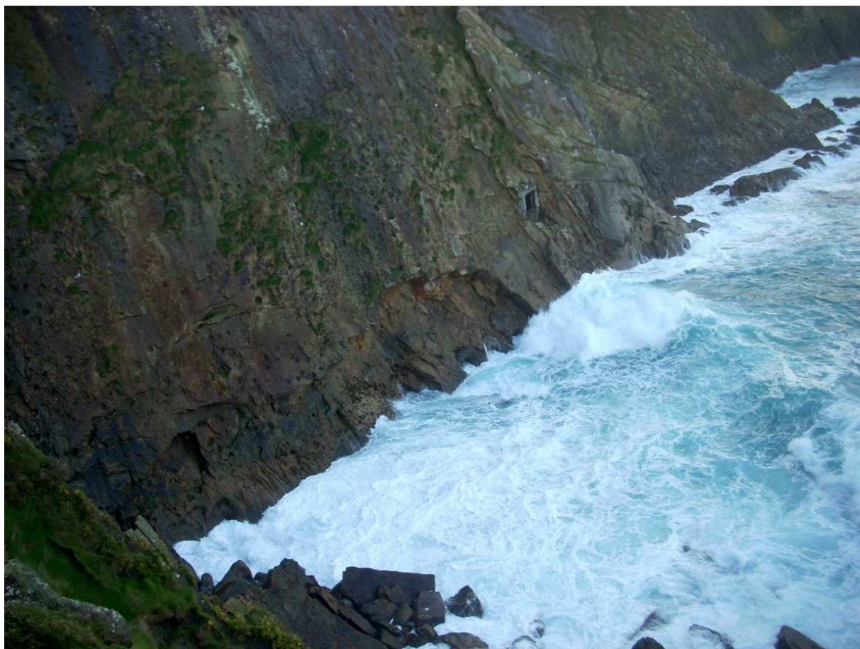
Figura 5. Punta W de Bajo aundi. Acantilado frontal (imagen superior) y playa de bloques casi cubiertos por la marea alta en su flanco W. Se aprecia la salida de una galería artificial rectangular y 4 aliviadores tubulares a nivel del mar del sistema de desagüe del colector submarino de Ulía. Nótese la fractura del estrato por erosión de su parte basal. Las imágenes son con marea alta. Durante la bajamar puede accederse a una pequeña playa de bloques de colapso.
