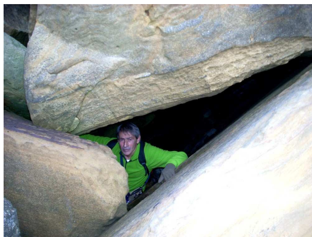
Figura 11. Cueva entre estratos de arenisca en la punta central de Bajo aundi, con recubrimiento de bloques. La claridad próxima en las imágenes se debe al flash, correspondiendo la luz natural sólo a las bocas, situadas al fondo de las imágenes.
