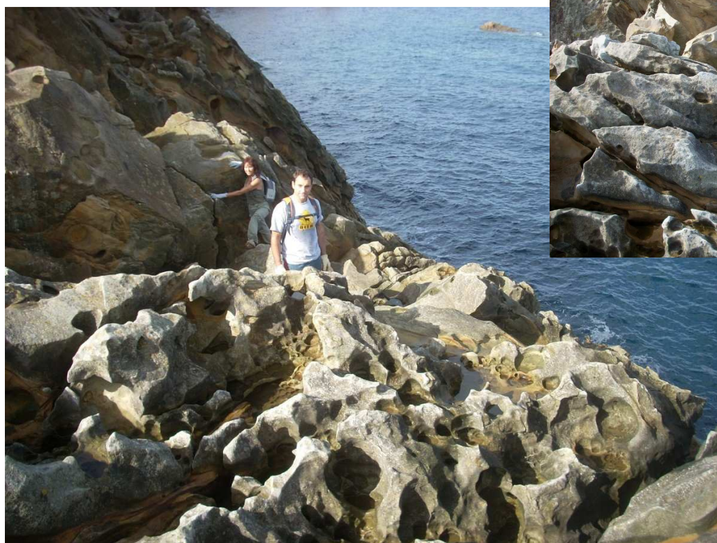
Figura 4. Prospecciones en la punta oriental de Bajo aundi; al fondo la punta central con dos cuevas interestratos en su flanco Este (imagen superior). Detalles de erosión marina con cubetas y geoformas de tipo lapiaz.
