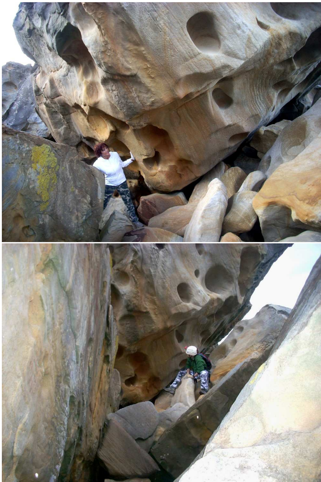
Figura 13. Promontorio de la punta central, con grandes bloques, bajo los cuales se desarrolla una cueva de 80 m. La boca superior (B1) se localiza detrás del espeleólogo de la imagen inferior.
