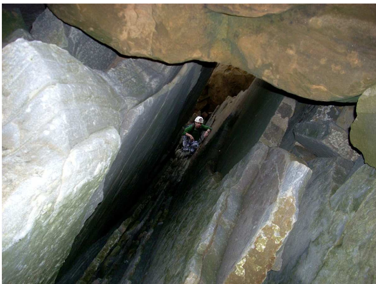
Figura 10. Cueva interestratos de caliza arenosa, en la punta central. La erosión pluvial y marina ha desgastado los estratos delgados de lutitas y margas. Grandes bloques de arenisca recubren el techo. Las fotos han sido tomadas desde la parte central oscura hacia ambos extremos (la luz de los planos próximos es del flash de la cámara).
