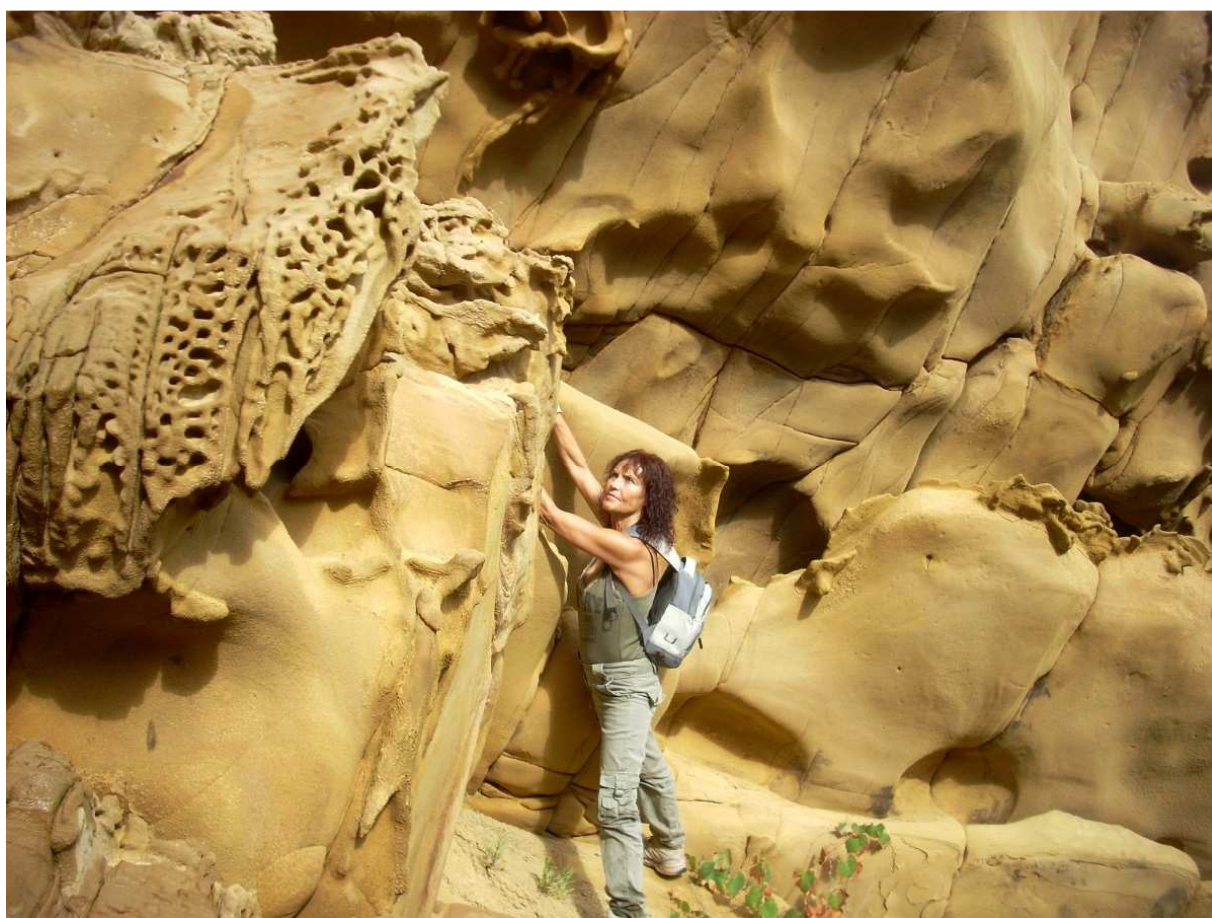
Figura 3. Roca amenizada por disolución intergranular, con cavidades y geoformas en los flancos extraplomados de los espolones de la punta E de Bajo aundi.
