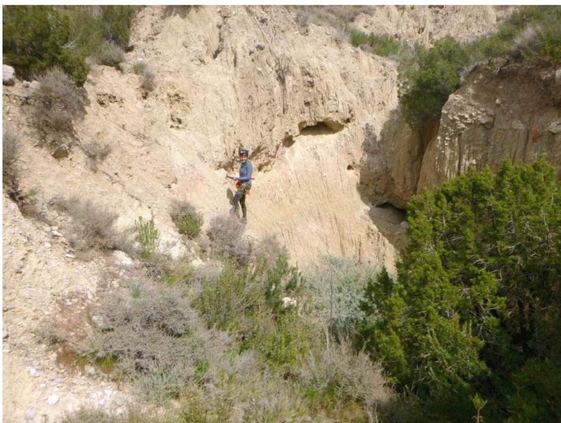
Figura 23. Sector Norte (arriba) y Sur (debajo) de la Sima Tripa Azul 03 (onceava cavidad), localizada en un zanjón cerrado de trazado complejo. La depresión-sima tiene 20 m de largo y hay que bajar por distintos puntos para explorar sus diversas zonas bajas internas. La mayor de ellas tiene una galería de 54 m y la sima en conjunto totaliza 91 m.
