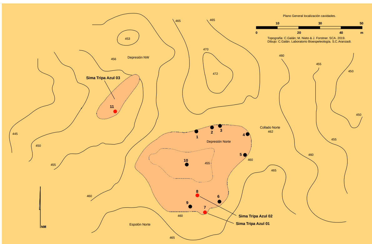
Figura 01. Imagen de satélite del espolón N de Tripa Azul (visto desde el N) con la localización de cavidades (arriba). Fuente imagen: Google Earth. Plano esquemático de ubicación de cavidades en la depresión del collado N (debajo).
