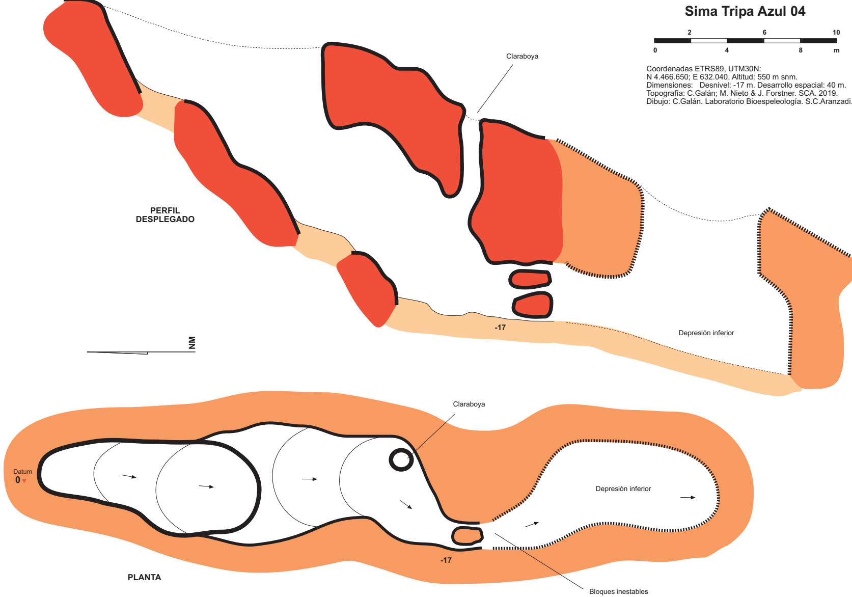
Figura 35. Plano de la sima 04.
