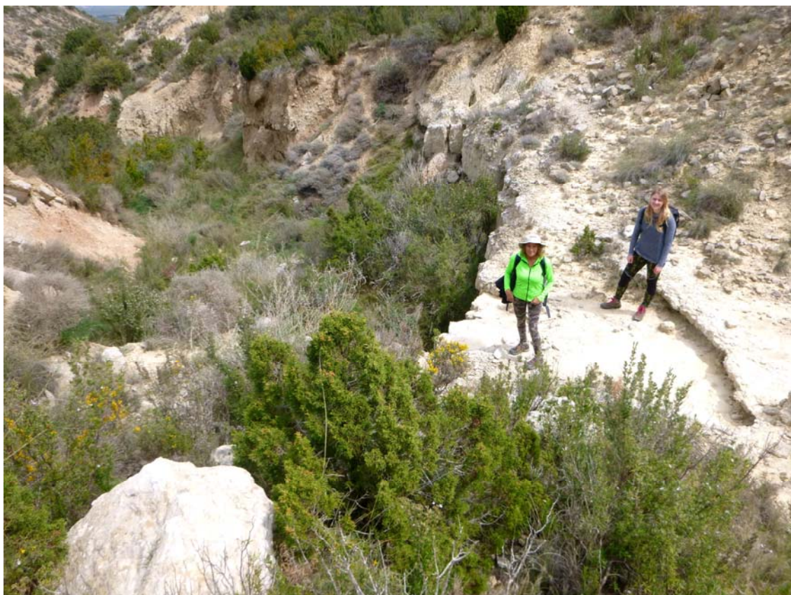
Figura 03. Solapa rocosa de margas en la cota 430 m snm de talweg del barranco de Tripa Azul.
