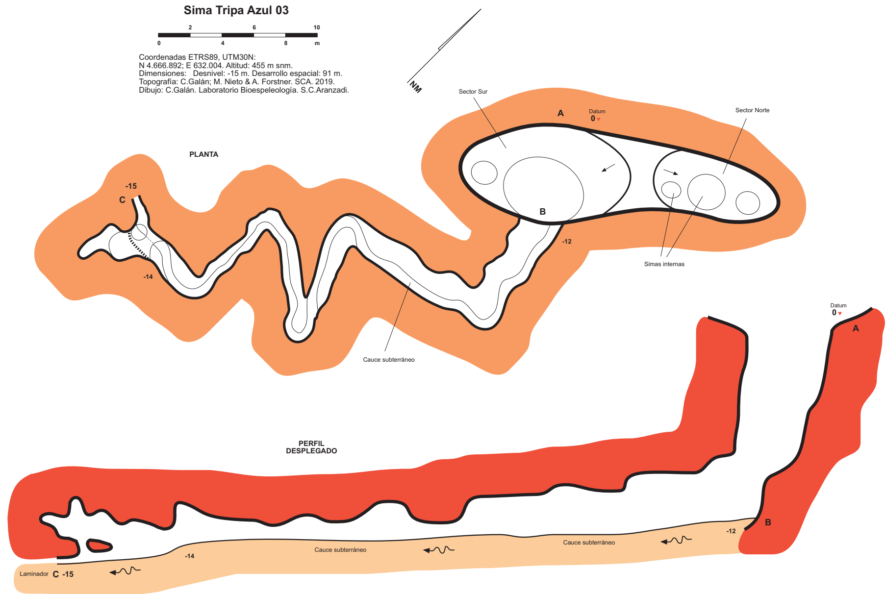
Figura 34. Plano de la sima 03.
