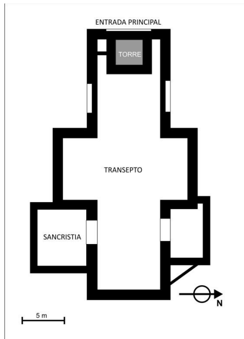
Planta da Igrexa de Flariz
