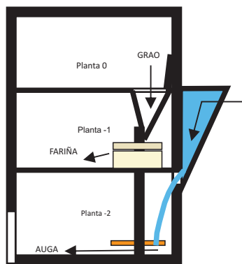
MUIÑO DA TRAPA Sección
