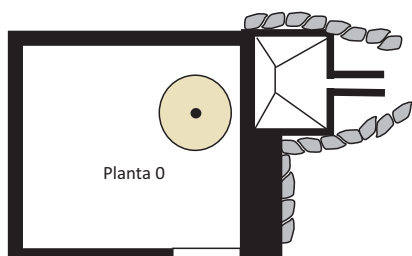
MUIÑO DO TOXAL Planta
