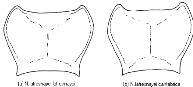
3. Irudia.- Nebria lafresnayeri pronotoak. Figure 3.- Nebria lafresnayeri pronotum.
