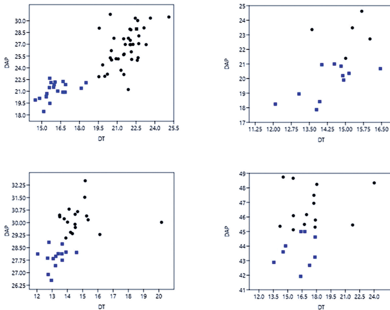
Fig.6. Dimorfismo sexual en la dentición superior de los Ursus spelaeus adulto de la cueva de Oilaskoa. Arriba de izquierda a derecha ( C^5 , P^4 ) abajo ( M^1 y M^2 ), los puntos azules representan a las hembras y los negros a los machos. En el análisis han sido considerados el Diámetro transversal (DT) y Diámetro anteroposterior (DAP) de cada una de las piezas (información biométrica, tabla A1 de los anexos). / Sexual dimorphism in the upper dentition of adult Ursus spelaeus from Oilaskoa cave. Above from left to right ( C^5 , P^4 ) below ( M^1 and M^2 ), the blue dots represent the females and the black dots represent the males. The analysis have considered the Transverse Diameter (DT) and Anteroposterior Diameter (DAP) of each of the teeth (biometric data in the annexes, table A1).
