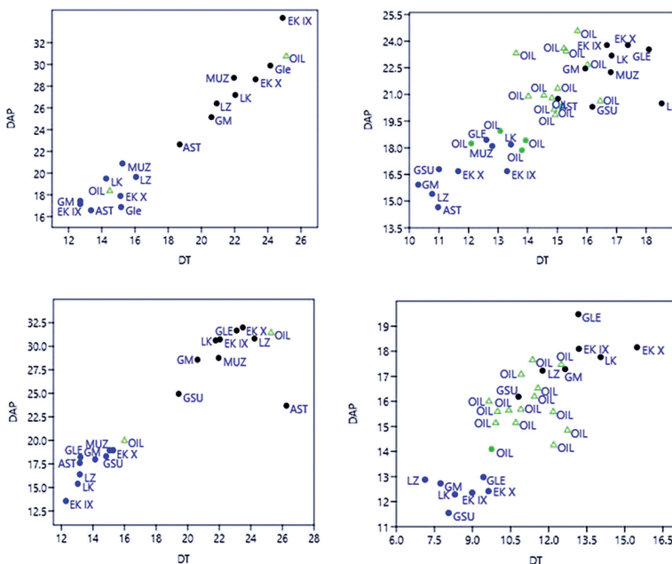
Fig.7. Análisis comparativo del Canino superior (C S ), cuarto premolar superior (P 4 ) ambos arriba y Canino inferior (C 1 ) y cuarto premolar inferior (P 4 ) de los restos de Ursus spelaeus de Oilaskoa en comparación con otros conjuntos del cantábrico oriental (información biométrica Anexos A1, A2 y A3). / Comparative analysis of the upper canine (C S ), upper fourth premolar (P 4 ) both above and lower canine (C 1 ) and lower fourth premolar (P 4 ) of the remains of Ursus spelaeus from Oilaskoa in comparison with other assemblages from the eastern Cantabrian (biometric data Annexes A1, A2 and A3). GM: Mairulegorreta (Zigoitia, Álava-Araba), GLE: Cueva de Legorras (Zigoitia, Álava-Araba), GSU: Cueva de Sugusti (Zigoitia, Álava-Araba), LZ: Lezetxiki (Arrasate, Gipuzkoa), AST: Astigarragako Koba (Deba, Gipuzkoa), LK: Labeko Koba (Arrasate, Gipuzkoa), MUZ: Muniziaga (San Pedro de Galdames, Bizkaia), EK: Ekain (Deba, Gipuzkoa).
