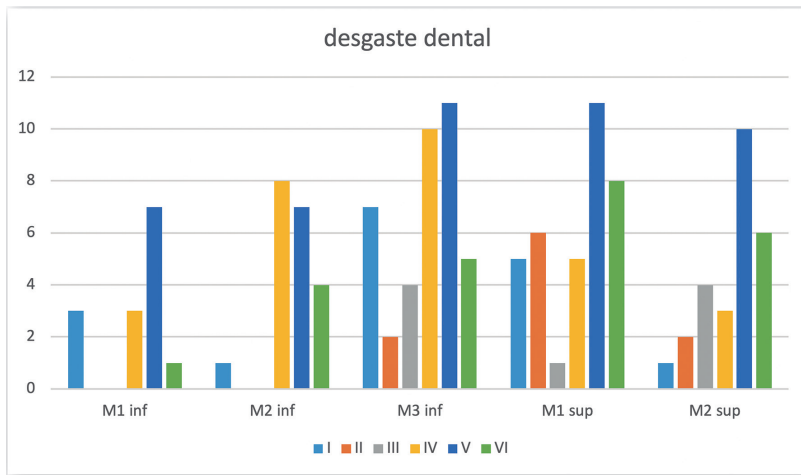
Fig.4. En la siguiente gráfica se muestra el desgaste dental documentado en los molariformes. Nótese la menor frecuencia de ejemplares subadultos o adultos jóvenes (I, II, III) frente a ejemplares de avanzada edad (V, VI), produciéndose el mayor pico de mortandad en la cohorte V. (ver tabla 7) / The following graph shows the documented dental wear in the molariforms. Note the lower frequency of subadult or young adult specimens (I, II, III) compared to elderly specimens (V, VI), cohort V documents highest mortality (see table 7).
