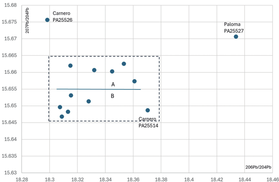
Fig.4. Comparación directa de todos los análisis de isótopos de plomo realizados a los metales del Museo de Amposta. / Direct comparison of all lead isotope analyses carried out on metals from the Amposta Museum.
